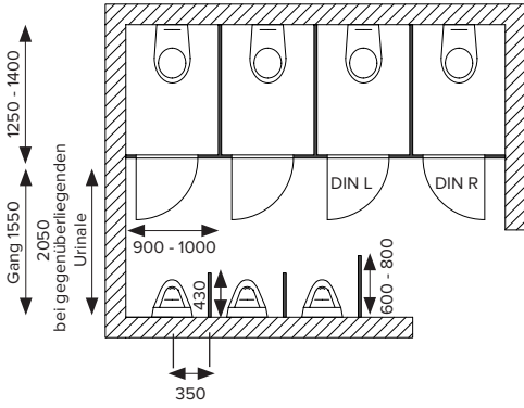
WC-Kabinen gegenüberliegend, Türen nach außen
