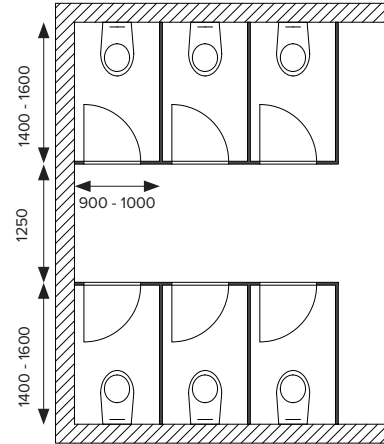
WC-Kabinen gegenüberliegend, Türen nach innen
