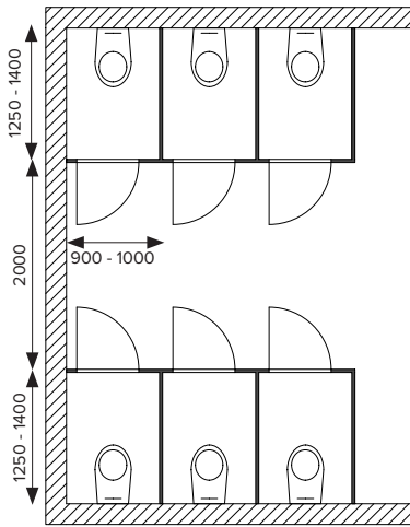
WC-Kabinen gegenüberliegend, Türen nach außen
