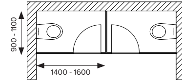
WC-Kabinen querliegend, Türen nach innen
