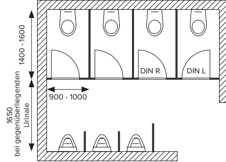
WC-Kabinen, Türen nach innen, Schamwände, Sichtschutzwände
