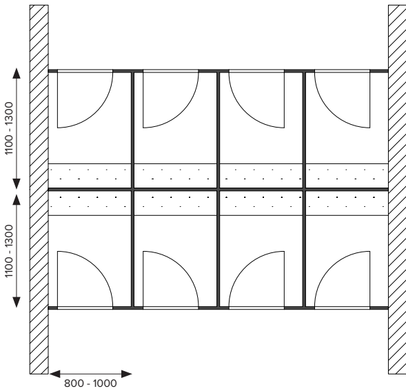
Umkleidekabinen doppelreihig, Türen nach innen
