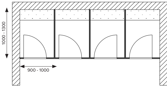
Umkleidekabinen, Türen nach innen
