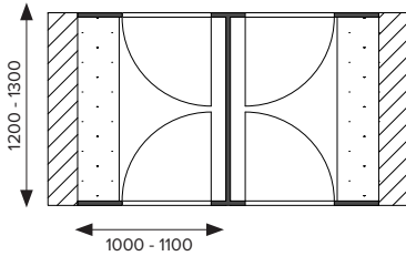
Wechselkabinen mit Zentralverriegelung, Türen nach innen
