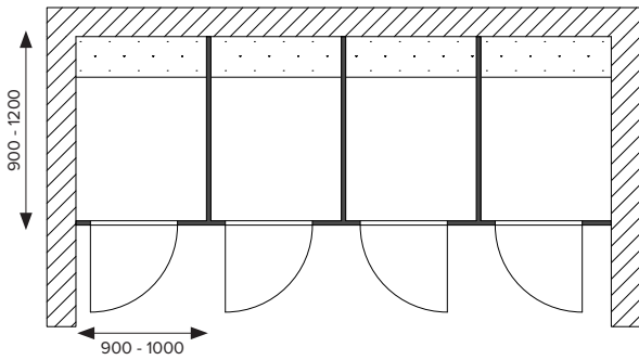
Umkleidekabinen, Türen nach außen
