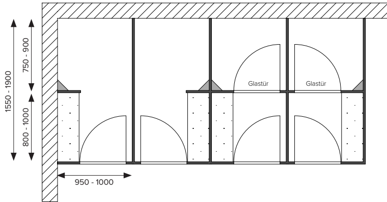
Duschkabinen mit Umkleibereich, Türen nach innen
