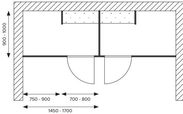
Duschkabinen mit Umkleibereich, Querliegend mit Türen nach außen
