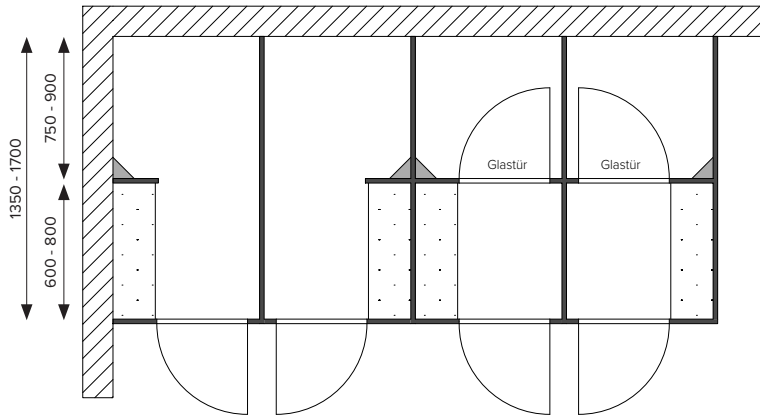
Duschkabinen mit Umkleibereich, Türen nach außen
